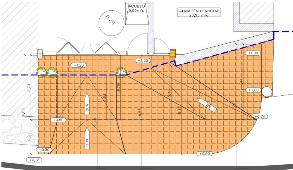
Figure 5: Acotado de la nueva alineación de fachada oeste.
